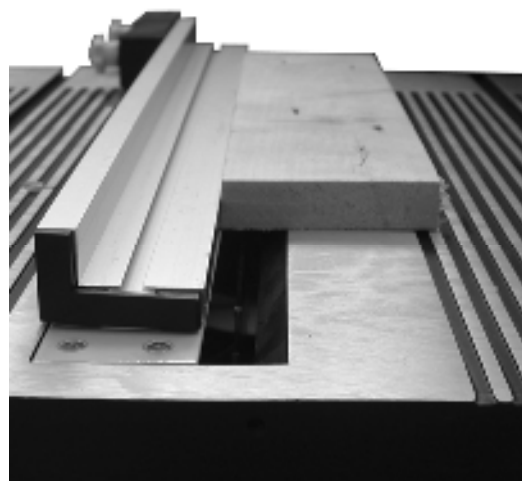
Рис. 21. Обработка низких и фасонных заготовок.
