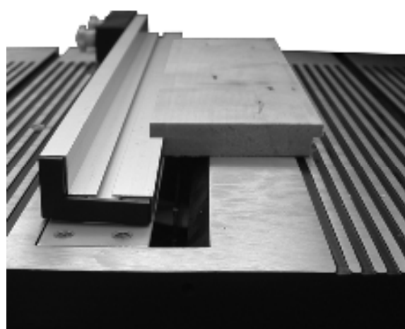
Рис. 21. Обработка низких и фасонных заготовок.
