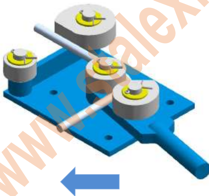
Прут, согнутый при помощи гибочных машин DR-25
