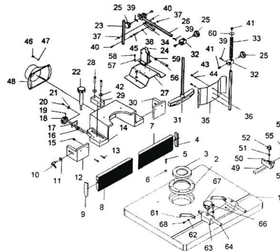
ДЕТАЛИ СБОРКИ ФРЕЗЕРНОГО СТАНКА «КОРВЕТ 84»
